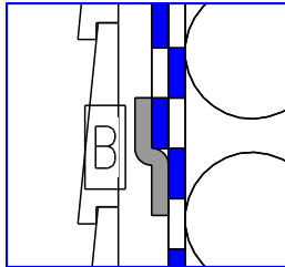
SIGA-Majcoat, verklebt mit SIGA-Wigluv
