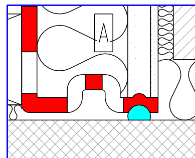
Luftdichter Anschluss auf Betonboden mit SIGA-Primur
