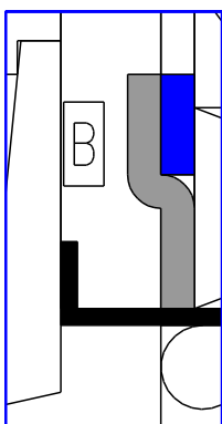
Winddichter Anschluss mit SIGA-Wigluf
