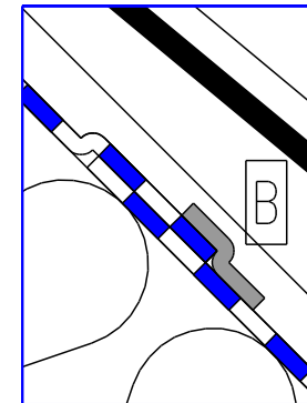
Überlappung, winddicht verklebt mit SIGA-Wigluf
