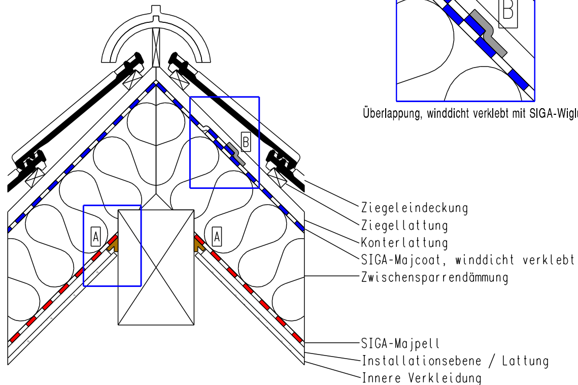
Luftdichter Anschluss an Firstpfette mit SIGA-Corvum 30/30
