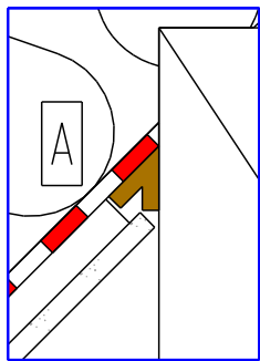
Luftdichter Anschluss an Firstpfette mit SIGA-Corvum 30/30
