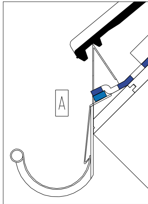
Anschluss SIGA-Majcoat auf Einlaufblech mit SIGA-Wigluv
