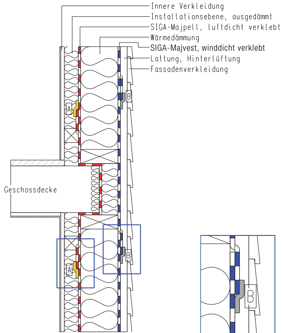
SIGA-Majvest, verklebt mit SIGA-Wigluv
