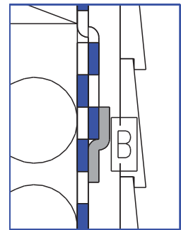
SIGA-Majvest, verklebt mit SIGA-Wigluv
